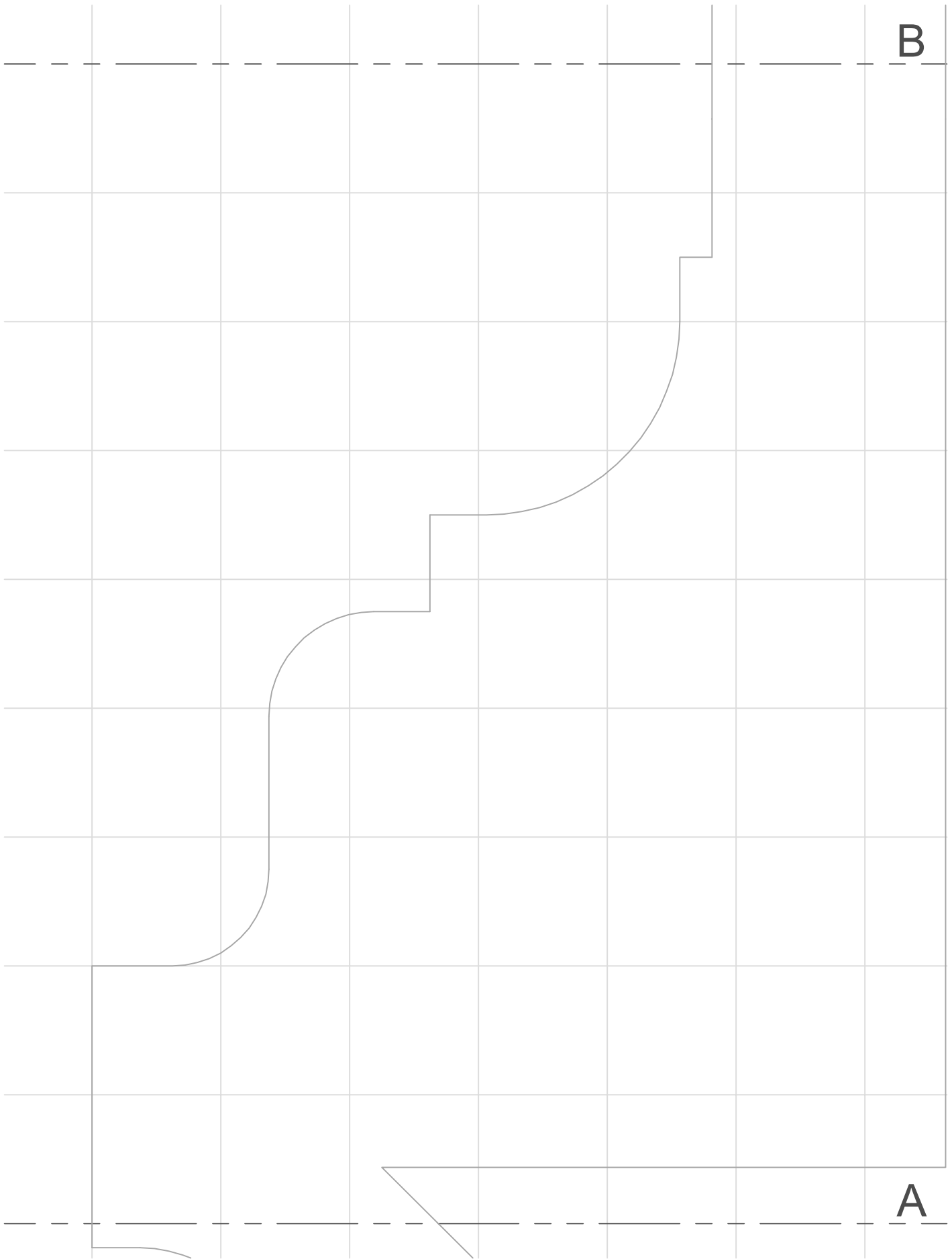
Front Apron - Sheet "B" Scale: 1" = 1"
