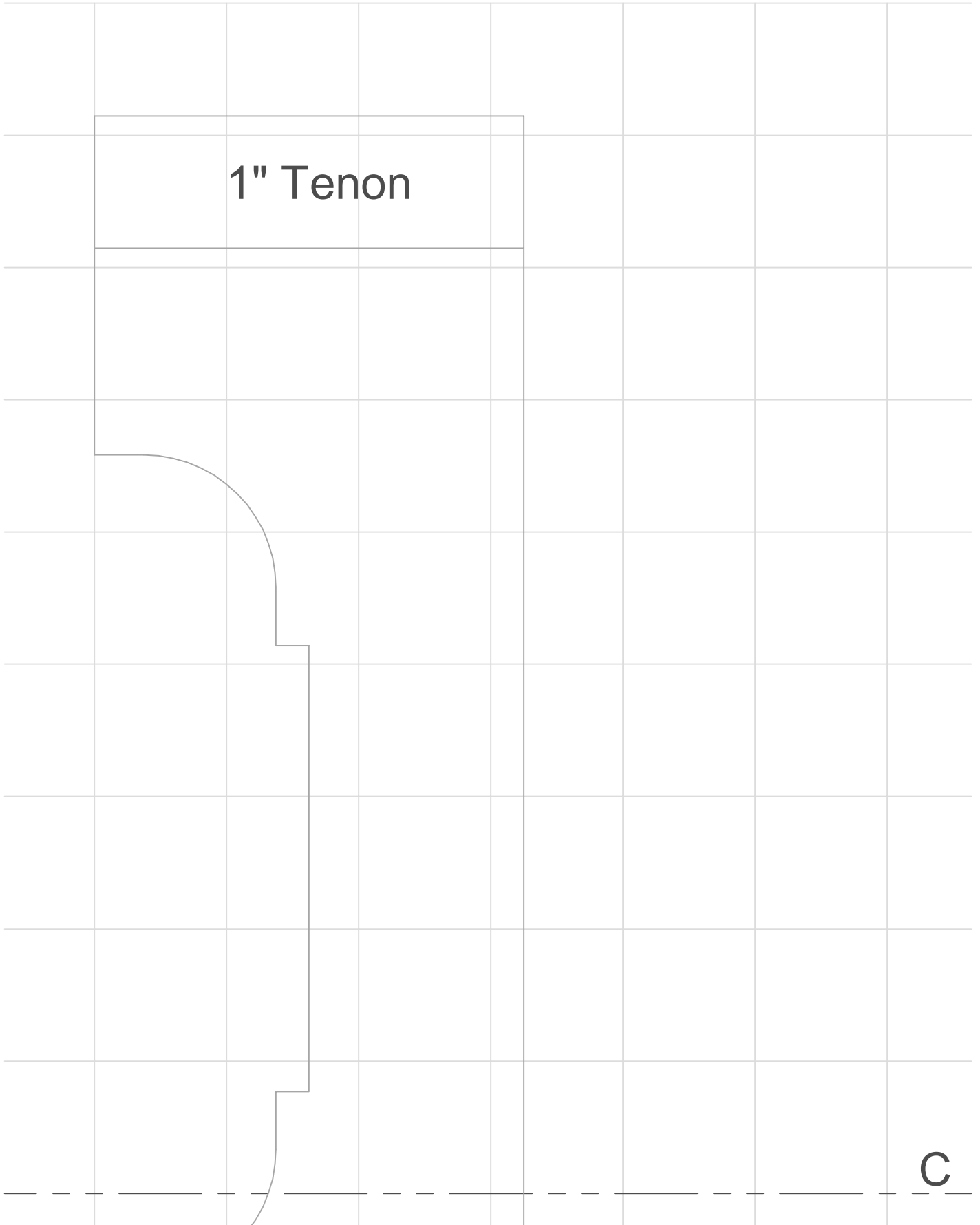
Front Apron - Sheet "D" Scale: 1" = 1"
